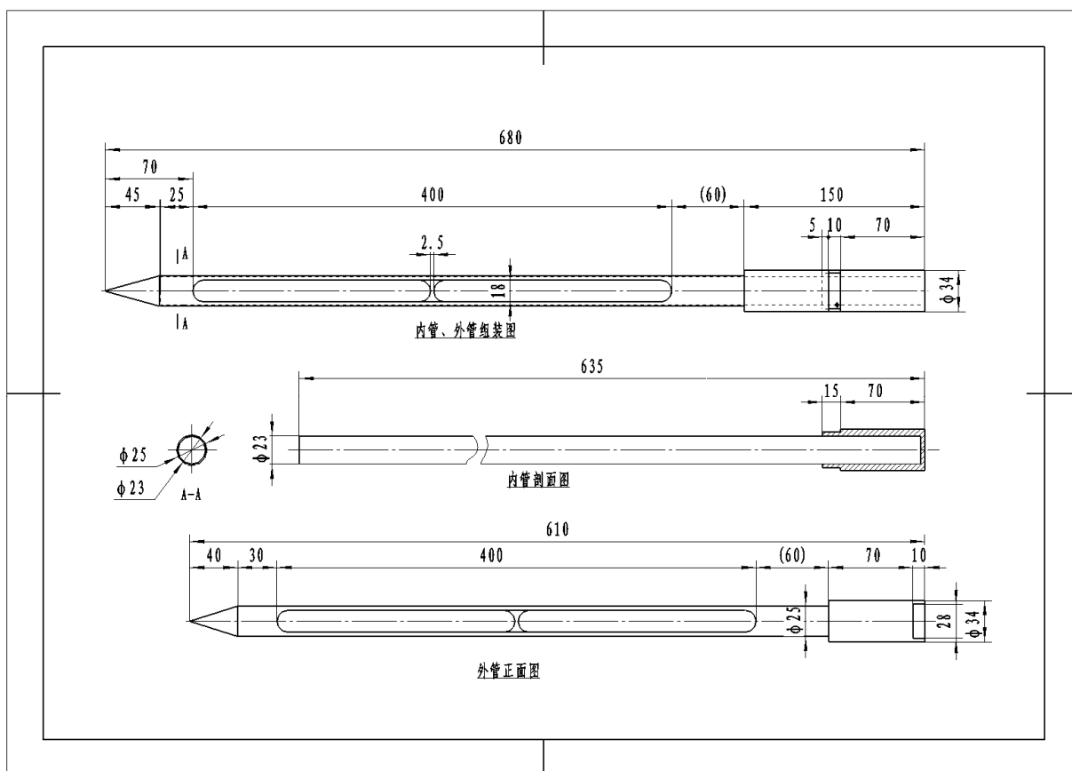
图1 采样探子
